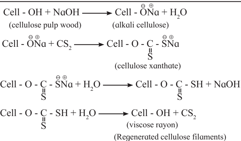
Fig. 15.7 : Formation of viscose rayon
